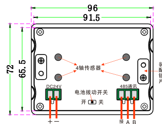
底视图 Bottom view
